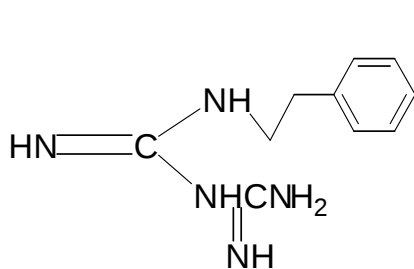
Phenformin ( 33 )
