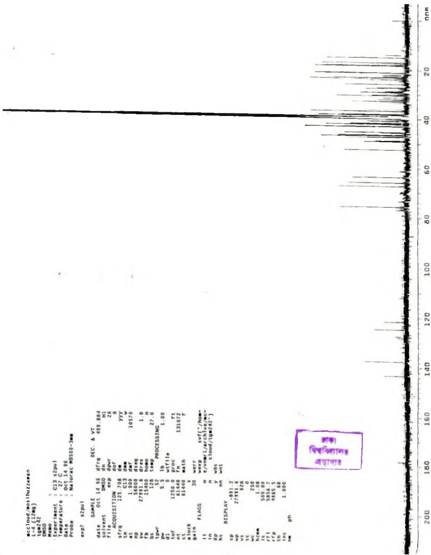
Fig 34 ^{13}\text{C} -NMR
