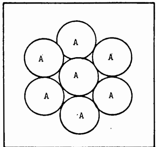
(d) Crystalline ( argon ( van der Waals )
