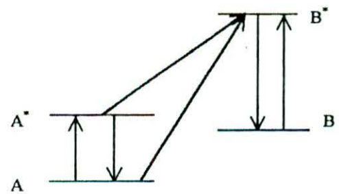
(d). Inelastic + Rearrangement, e.g. A(a, a')A^*(a', b)B
