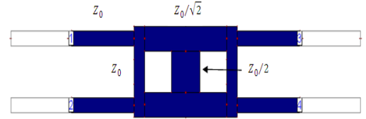
Fig. 3. Cross-coupler or 0dB coupler.
