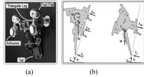
Fig. 4. Waalbot
