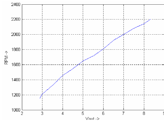
Fig. 5. Actual graph for V_{out} vs RPM
